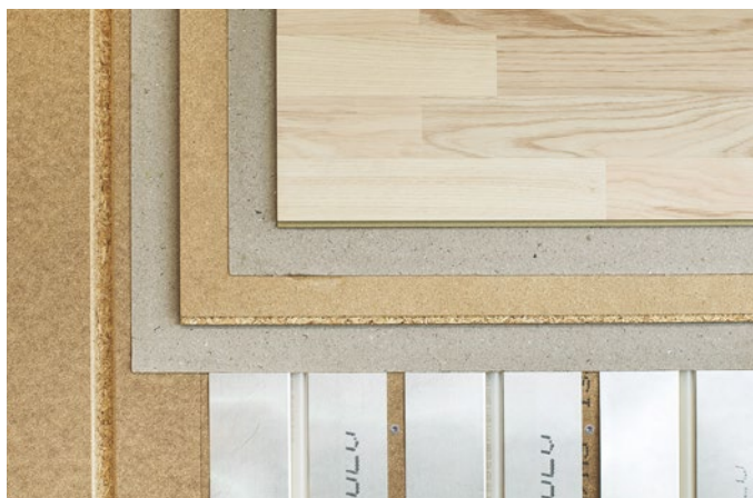
Figur 12 Der bør altid lægges gulvpap mellem varmfordelingsplader og undergulvsplader samt mellem undergulvsplader og trægulve for at hindre klapre- og knirkelyde.
