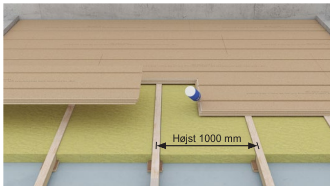
Figur 5 Klimagulv lagt i forbandt med flyvestød og pladeforskydning på mindst 450 mm. Må kun anvendes i almindelige boligrum.
